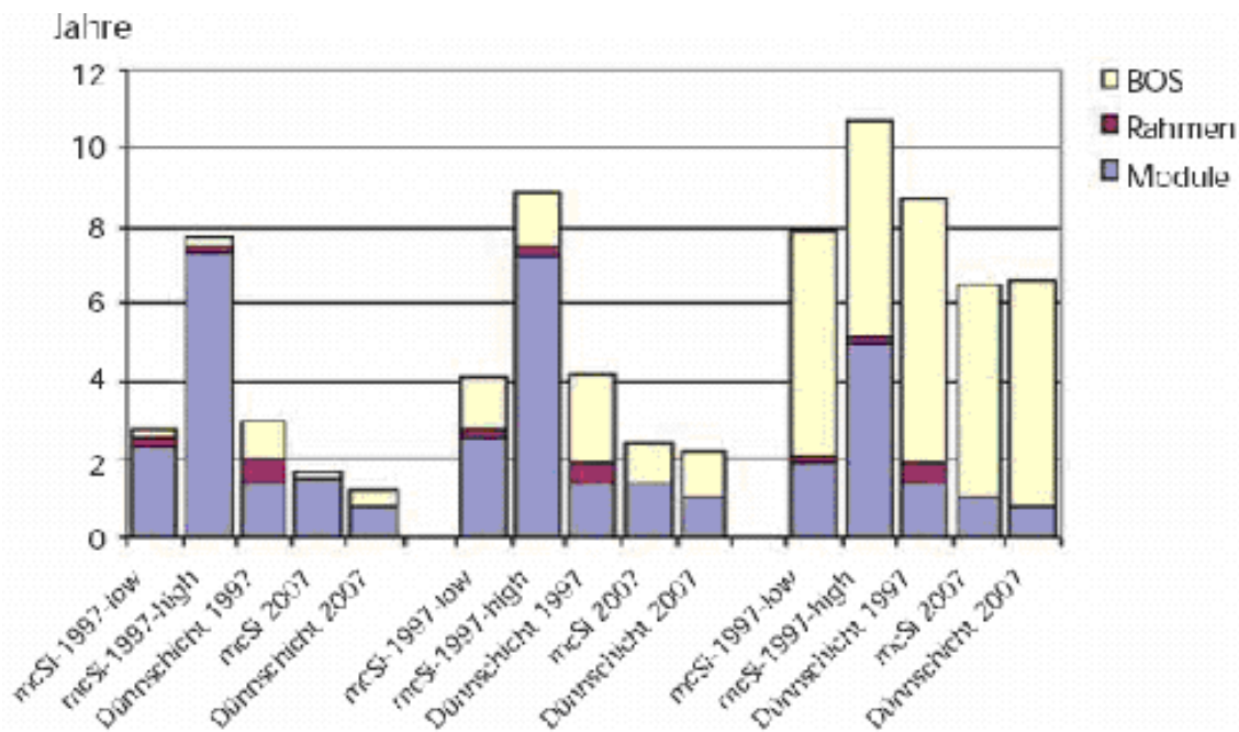
Abb. 8: Energierückgewinnungszeiten für Solarzellentypen (aus Springer 2003: 67) BOS sind die balance-of-system components, d.h. die nicht-photovoltaischen Teile der Solaranlage, wie Wechselrichter und Generatoren sowie bauliche Einrichtungen. „low“ steht für optimistische, „high“ für pessimistische Annahmen.
