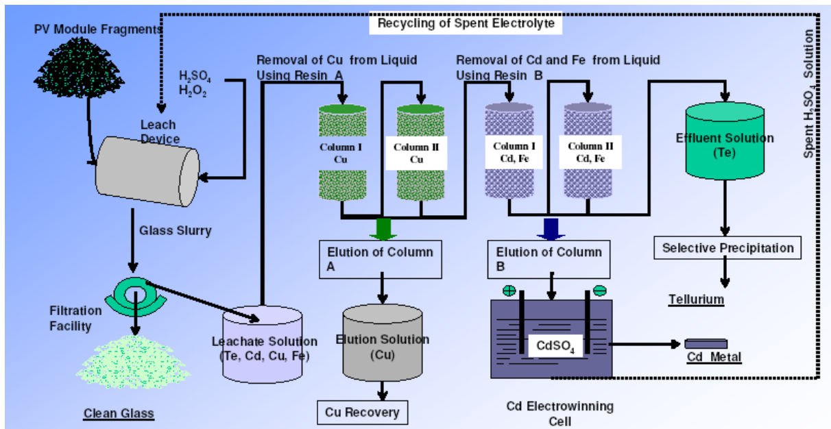
Abb. 53: Recycling von CdTe-Zellen (Alsema, de Wild-Scholten, Wambach 2007: 12)
