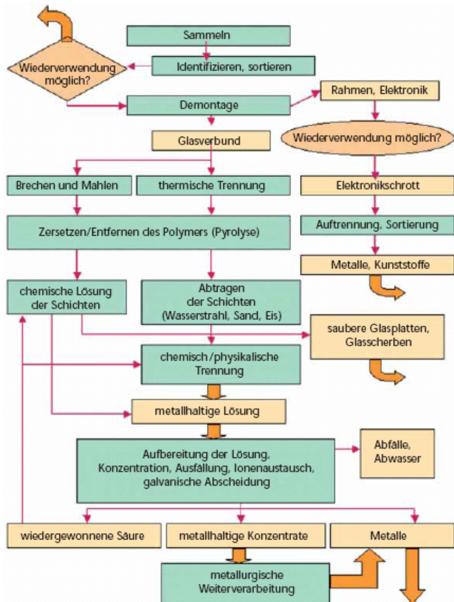
Abb. 52: Dünnschichtmodulrecycling (Springer 2003: 68)
