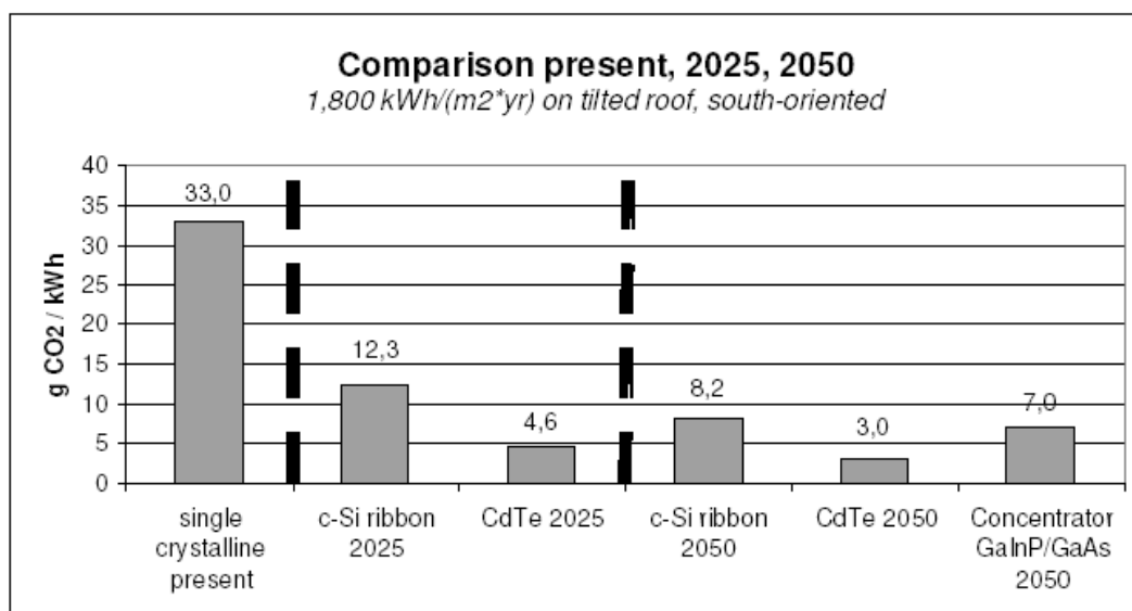
Abb. 19: Treibhausgasemissionen verschiedener Solarzellentypen (Raugei u.a. 2007: 18)
