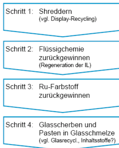
Abb.54: Recycling für Farbstoffsolarzellen ((Heubach 2007: 10)
