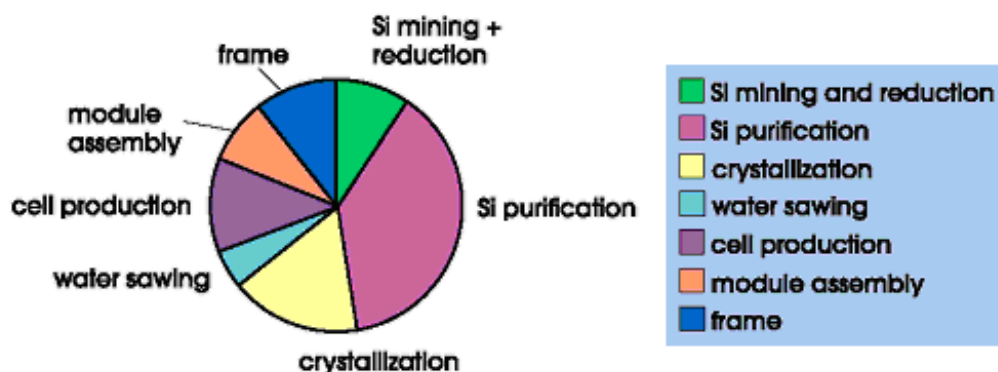
Abb. 6: Verteilung des Energieaufwandes für die einzelnen Herstellungsschritte (CrystalClear : 11) 7
