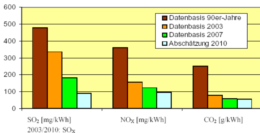
Abb. 27: Veränderungen aufgrund weiterer technischer Entwicklungen (Kruck, Eltrop 2007: 24)
