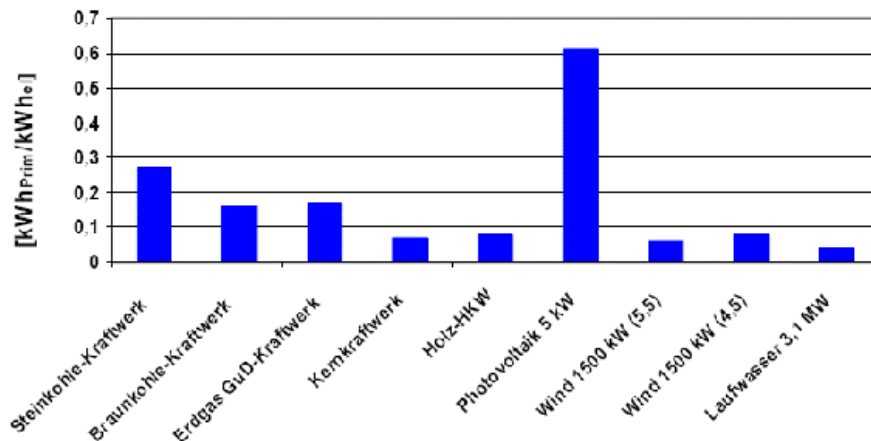
Abb. 12: Spezifischer kumulierter Energieaufwand 8 , ohne Einsatz des Brennstoffs (Voß 2008: 50, vgl. auch Mayer-Spohn u.a. 2006: 4) Wind unterschieden nach onshore (4.5) und offshore (5.5).
