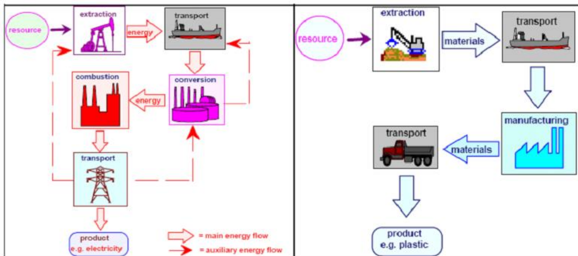
Abb.5: Life-Cycle-Analysen für Energieprodukte (links) und stoffliche Produkte (rechts) (Fritsche 2006: 2)
