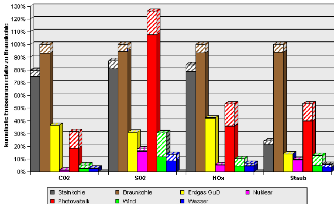
Abb. 25: Kohlendioxid-, Schwefeldioxid- und Stickoxid-Emissionen der Energieerzeugungstechniken der Energieerzeugungstechniken (aus Voß 2002: 16).
