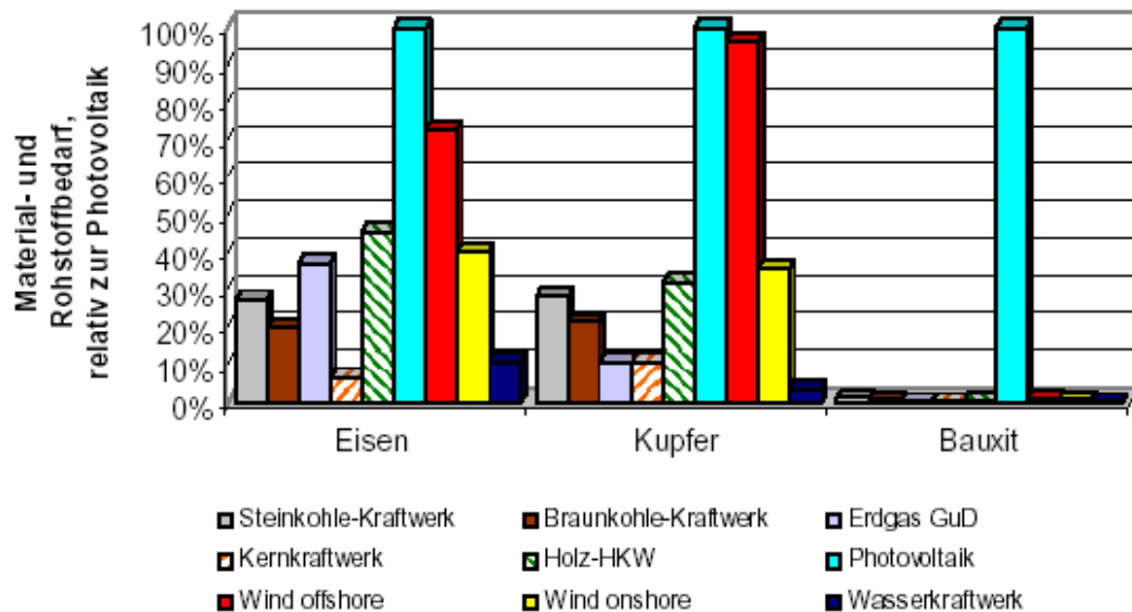
Abb. 33: Ressourcenverbrauch verschiedener Energieerzeugungsmethoden (Kruck, Eltrop 2007: 185)
