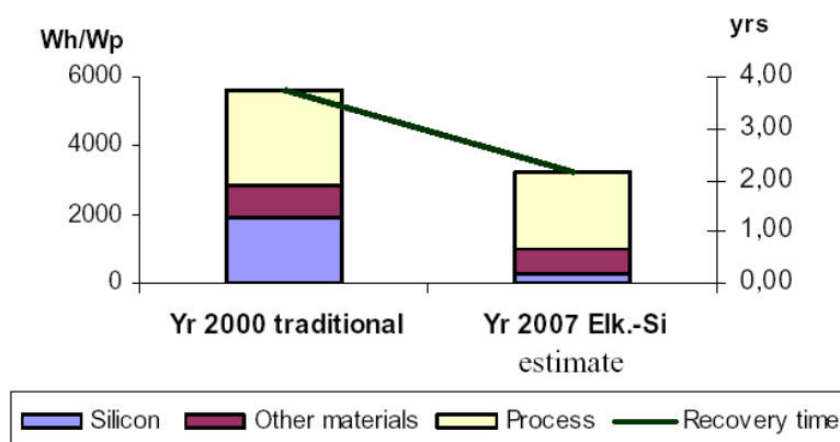
Abb. 10: Energieverbrauch und Paybackzeit bei Elkem-Silizium (Peter et al. 2005: 1)
