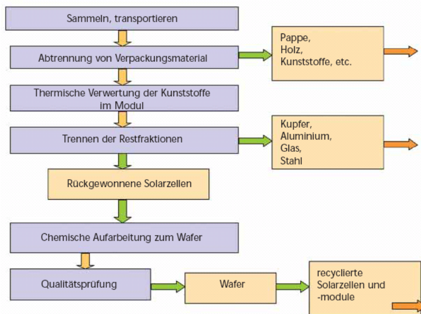
Abb. 51: Silizium-Wafer Solarmodulrecycling bei Solarworld (Springer 2003: 68)
