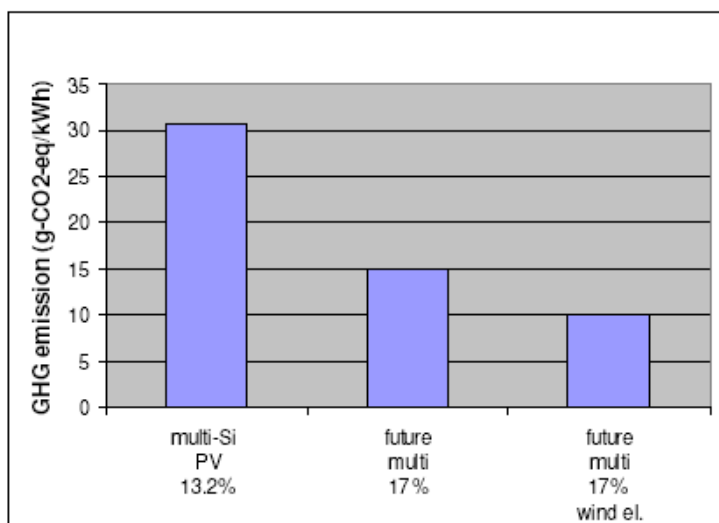
Abb. 18: Entwicklung der Treibhausgasemissionen von mc-Siliziummodulen (Alsema, de Wild-Scholten 2007a: 7)
