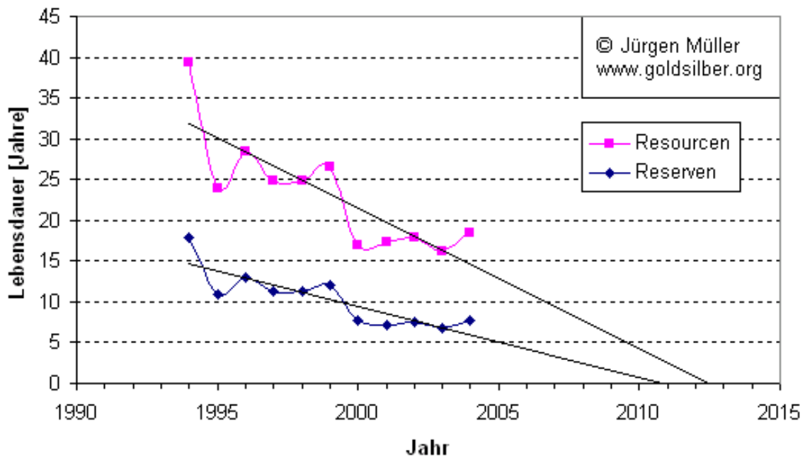
Bild 1: Extrapolierte Lebensdauern von Ressourcen und Reserven von Indium, (Quelle: USGS)
