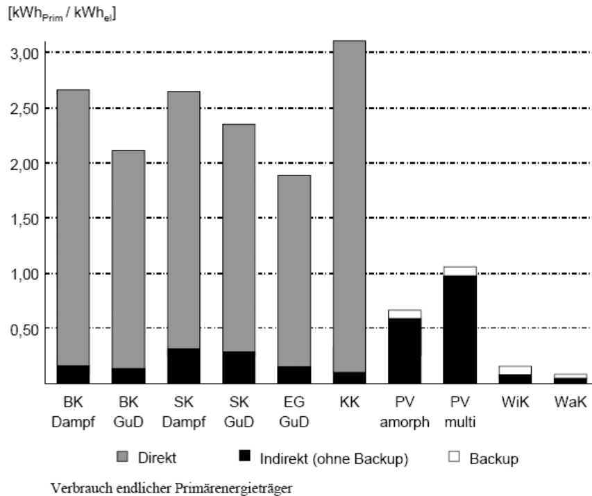
Abb. 13: Verbrauch endlicher Primärenergieträger (Marheineke 2002: 120). Die „direkten“ Anteile (grau) entsprechen dem Brennstoffeinsatz, indirekte Anteile enthalten z.B. auch den Transport der Steinkohle und das Backup bezieht sich auf zusätzliche Einrichtungen zur Speicherung der erneuerbaren Energie. (KK: Kernkraft, WiK: Windkraft, WaK: Wasserkraft)
