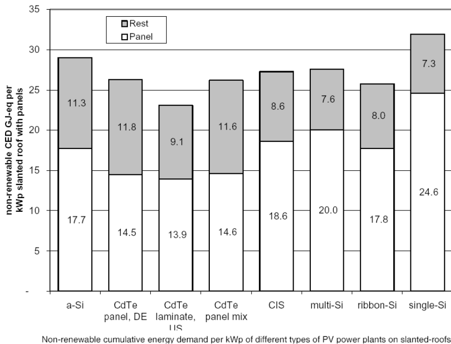
Abb. 11: Kumulativer (nicht erneuerbarer) Energieverbrauch (Jungbluth u.a. 2008: 12)
