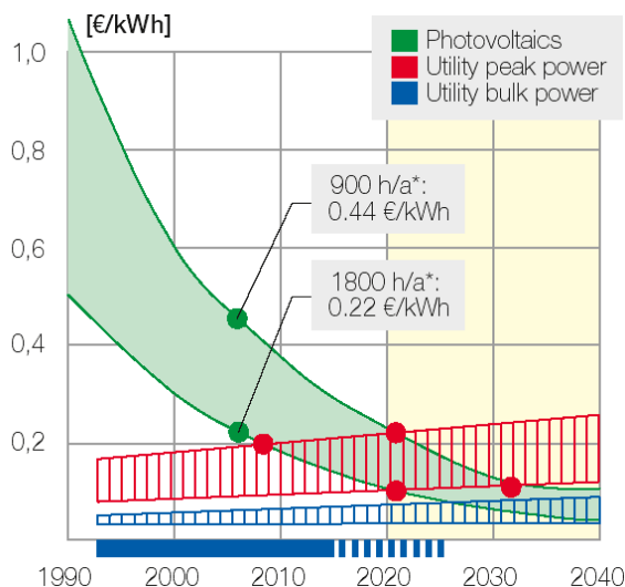
Abb. 1 Preissenkungstendenz in der PV („Lernkurve“) (aus EPIA, Greenpeace 2008: 41)
